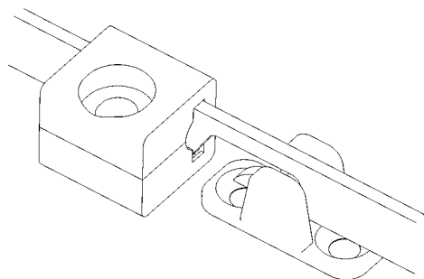
PARTICOLARE DI AGGANCIAMENTO ASTE RODS HOOKING VIEW STANGENKUPPLUNG
